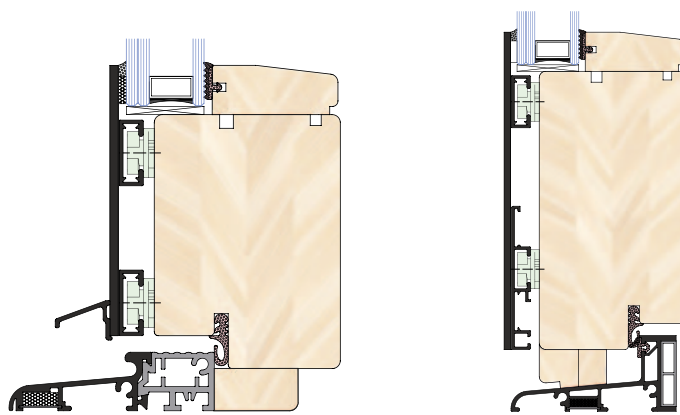
Inward opening door
