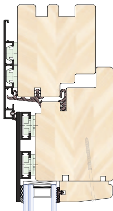
Door cross-section – top
